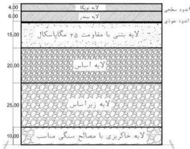
دیتایل فنی و اجرایی معابر بالای ۱۸ متر
